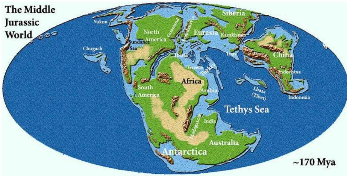
Die Welt im Jura mit ähnlichem (?) Klima wie heute (Mya = Mio Jahre) [6]
