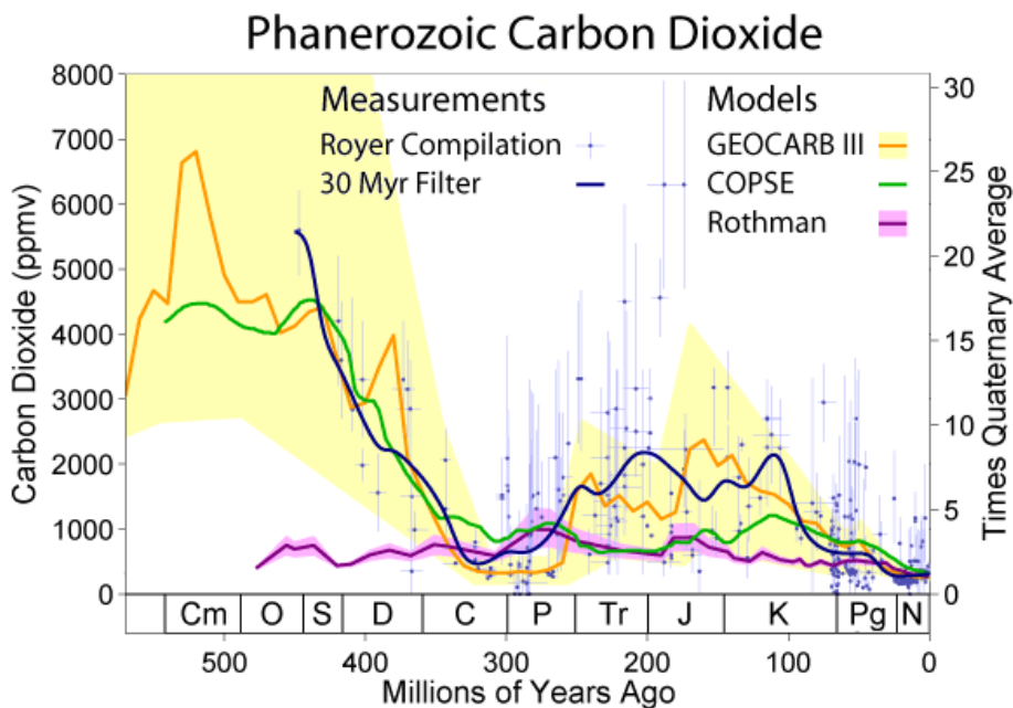
Jura, CO 2 (orange) zu „N“-Neuzeit [5]
